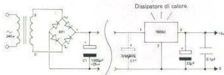
Fig. 6. Alimentazione addizionale +5V
